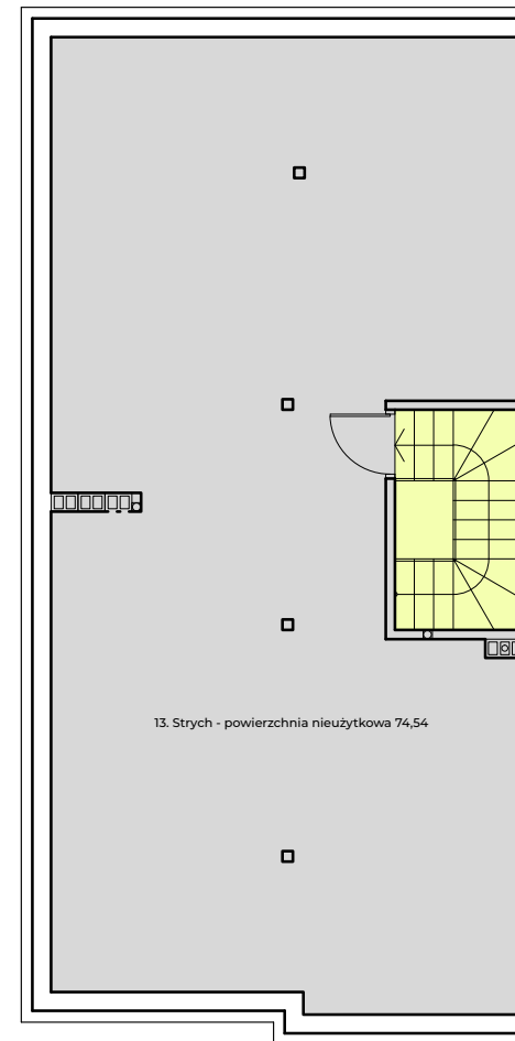
Poddasze
